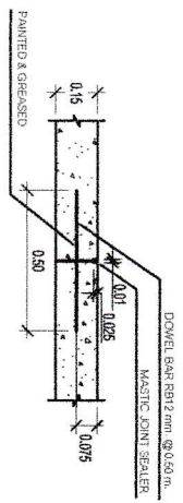
รอยต่อของจากากัดสราง Construction Joint มาตราส่วน 1 : 20
